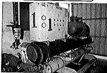
1號機kW/RT 改善前
