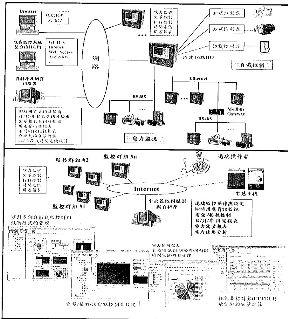
智慧節能系統架構(例)
